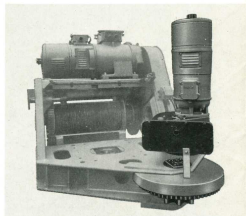
5 - Réducteur d'orientation ; moteur avec électro-frein.
