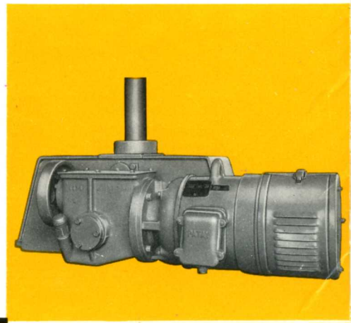
6 - Boggie moteur avec électro-frein.
