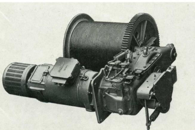
2 - Treuil de levage 3 vitesses avec frein à bande à commande électro-hydraulique et ralentisseur DYNAWEITZ
