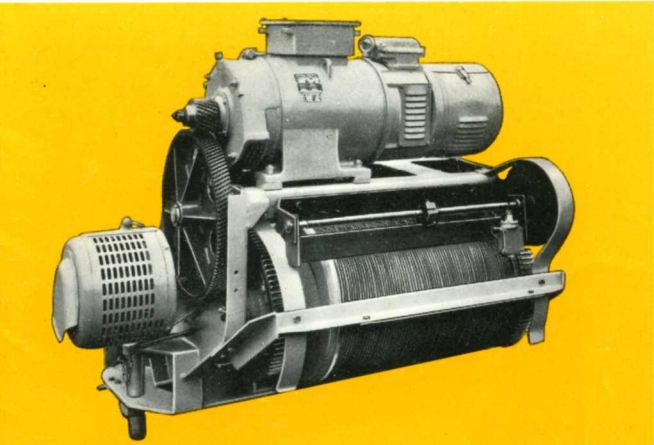
1 - Treuil de levage 2 vitesses avec électro-frein et ralentisseur DYNAWEITZ
