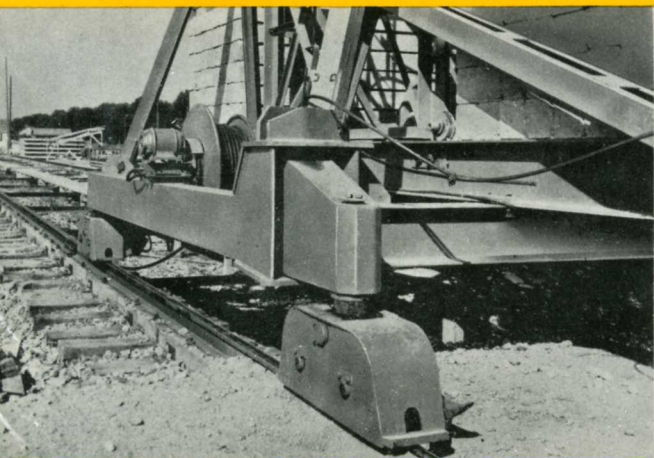
3 - Châssis avec boggies et bras articulés.
