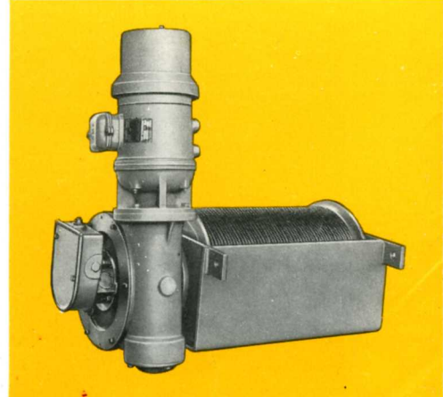
4 - Treuil de direction de chariot ; moteur avec électro-frein.
